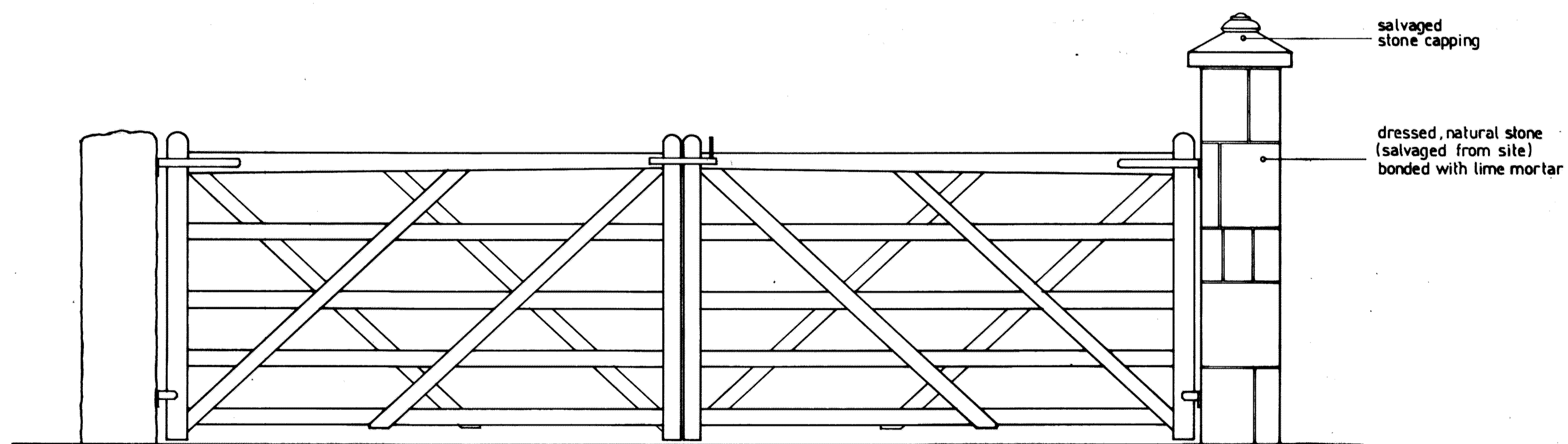
Gate(s) 3 Elevation 1:20
